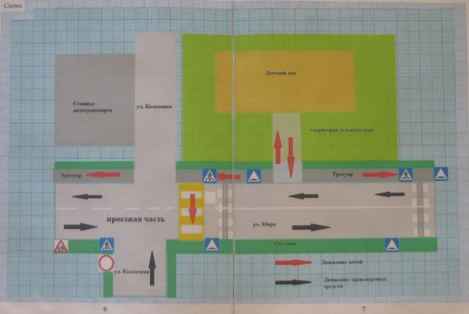
1.2. Схема организации дорожного движения в непосредственной близости от образовательной организации с размещением соответствующих технических средств, маршруты движения детей и расположение парковочных мест автотранспорта
